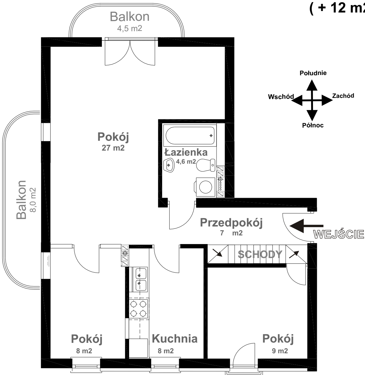
Pierwszy poziom - 3 pokoje 64 m 2
