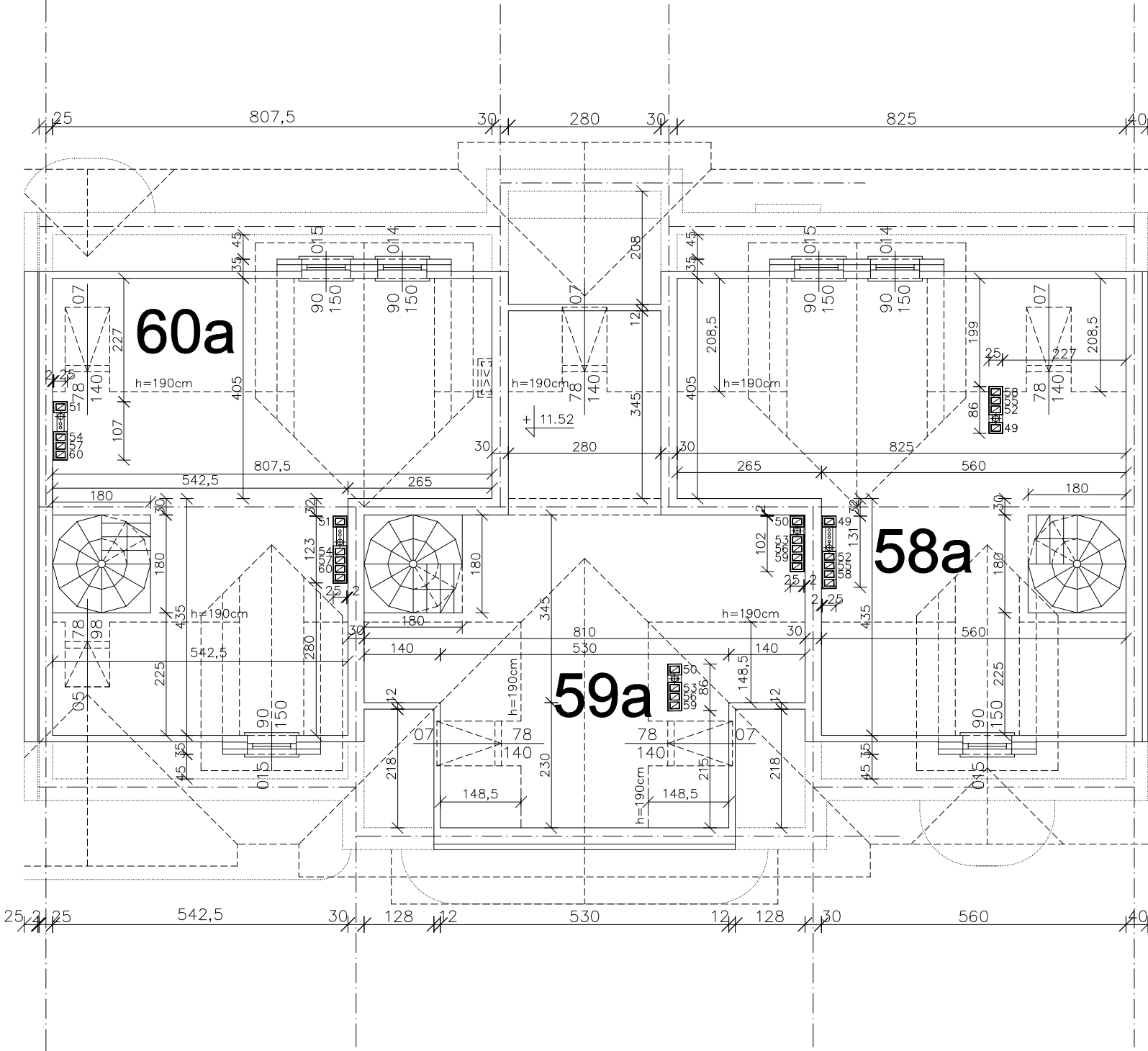
ZESTAWIENIE POWIERZCHNI UŻYTKOWYCH I PODŁÓG ANTRESOL – KLATKA V
